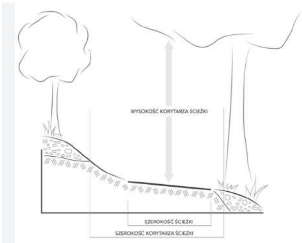
SCHEMAT 49. Przerznięcie równoważonej tras rowerowej.
