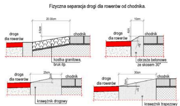
SCHEMAT 14. Przykładowa obniżenia drogi dla rowerów względem chodnika.
