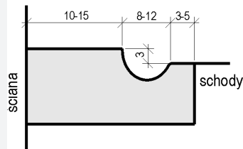
SCHEMAT 40. Kształt rampy kamiennej lub betonowej.
