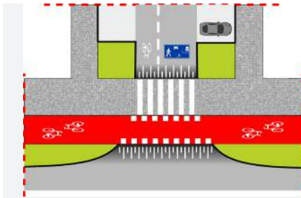
SCHEMAT 23. Wjazd bramowy.
