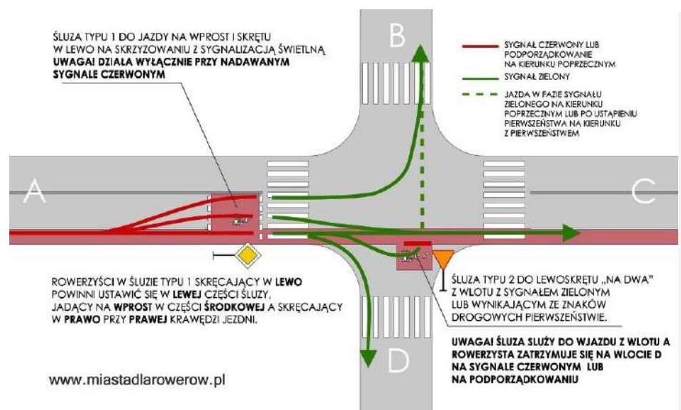
SCHEMAT 28. Rodzaje śluz rowerowych.
