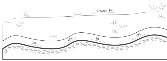
SCHEMAT 44. Średni spadek ścieżki wynosi 8%. Jednak chwilowe nachylenia są zmienne. Wprowadzenie odwróceń nachylenia powodują, że ścieżka naprzemiennie się podnosi i obniża.
