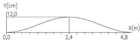
Profil wysokościowy progu sinusoidalnego – przekrój A-A
