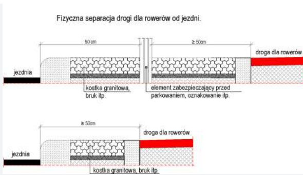
SCHEMAT 13. Przykładowa separacja drogi dla rowerów od jezdni.
