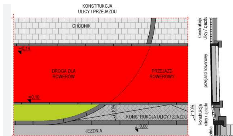
SCHEMAT 33. Przykładowe połączenie drogi dla rowerów z jezdnią.
