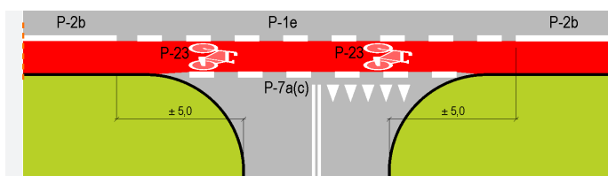
SCHEMAT 21. Przykład oznakowania pasa ruchu dla rowerów na skrzyżowaniu.
